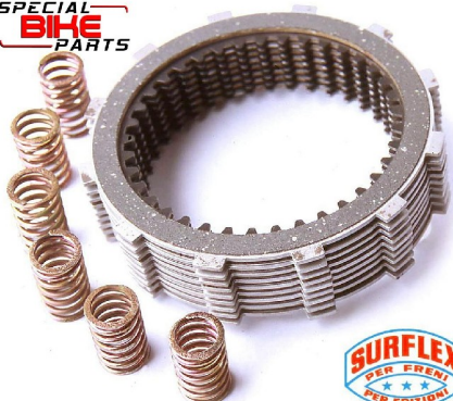
Kevlarmixbelag mit Druckfedern
